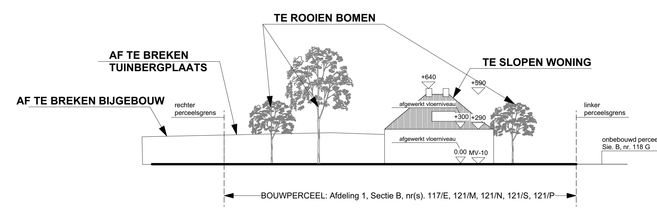
TERREINDOORSNEDEN 2 bestaande toestand schaal 1/200
