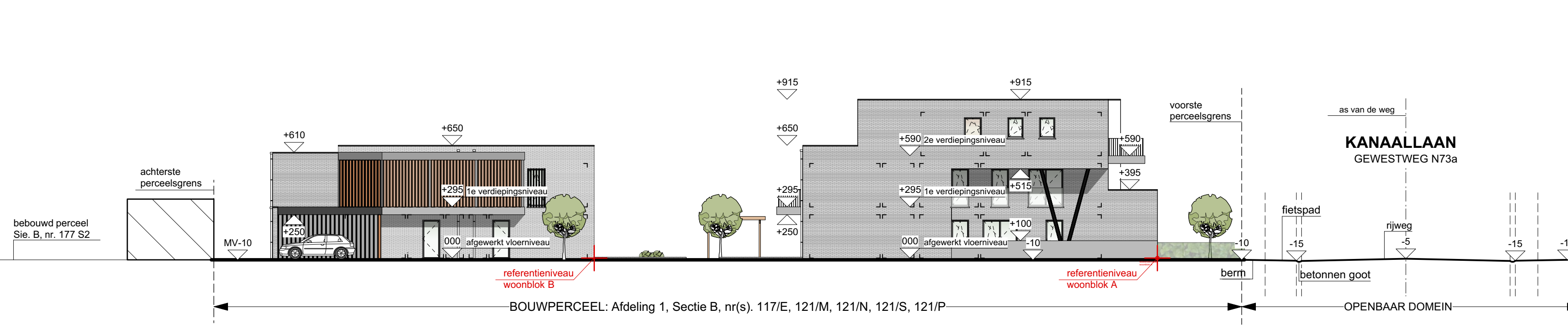
TERREINDOORSNEDEN 1 nieuwe toestand schaal 1/200
