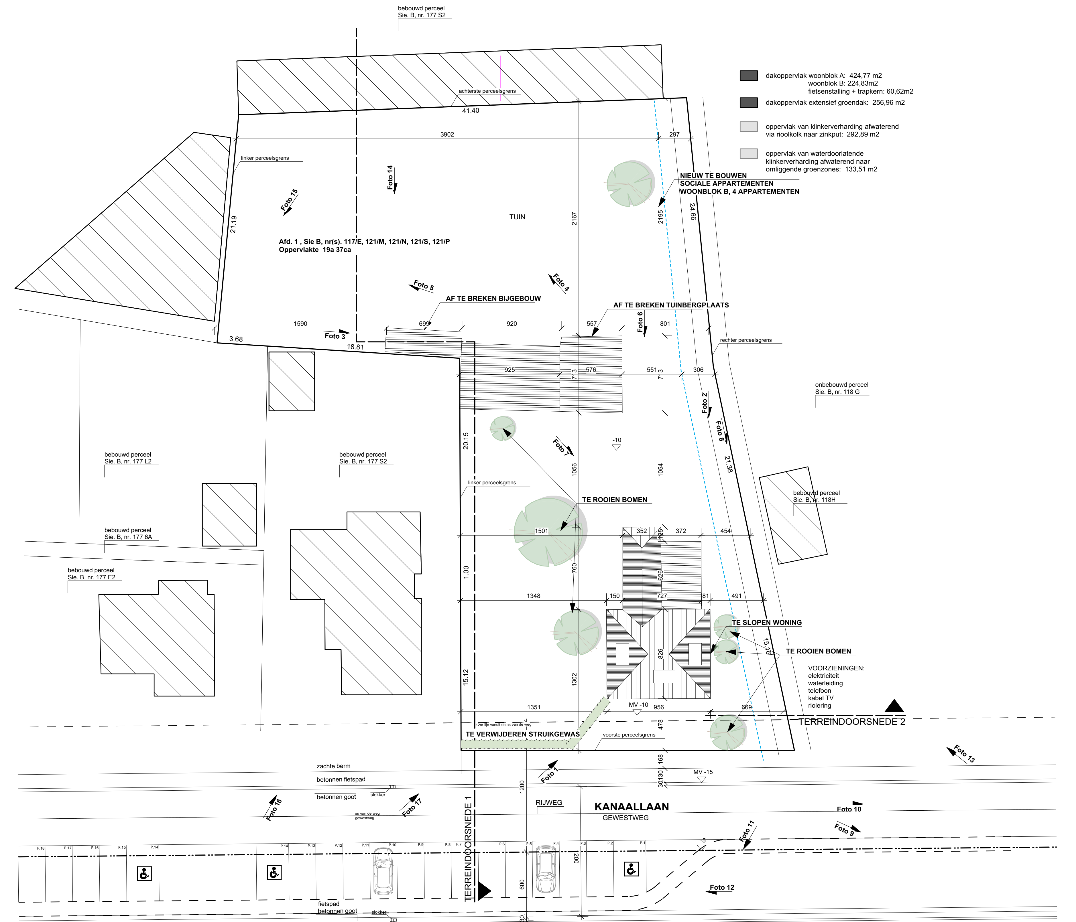
INPLANTINGSPLAN bestaande toestand schaal 1/200
