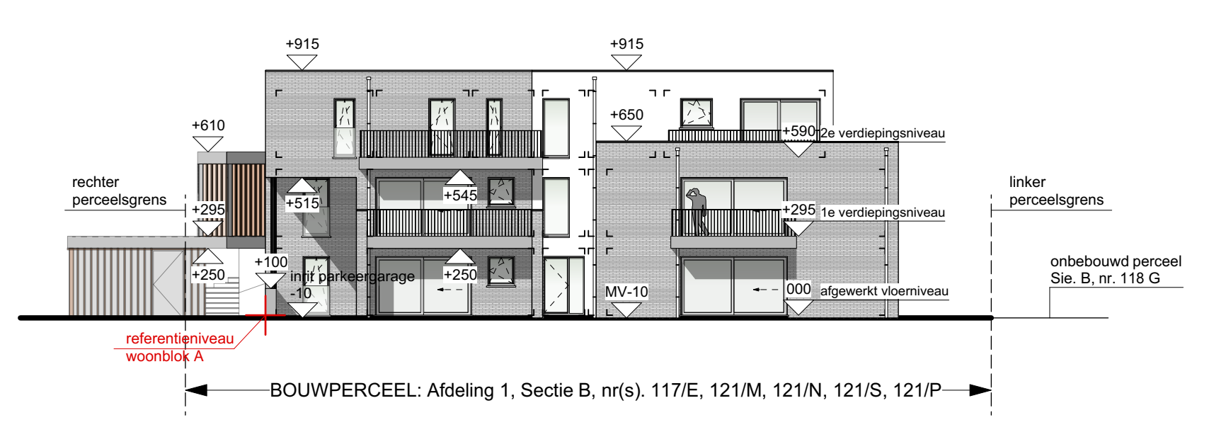
TERREINDOORSNEDEN 2 nieuwe toestand schaal 1/200
