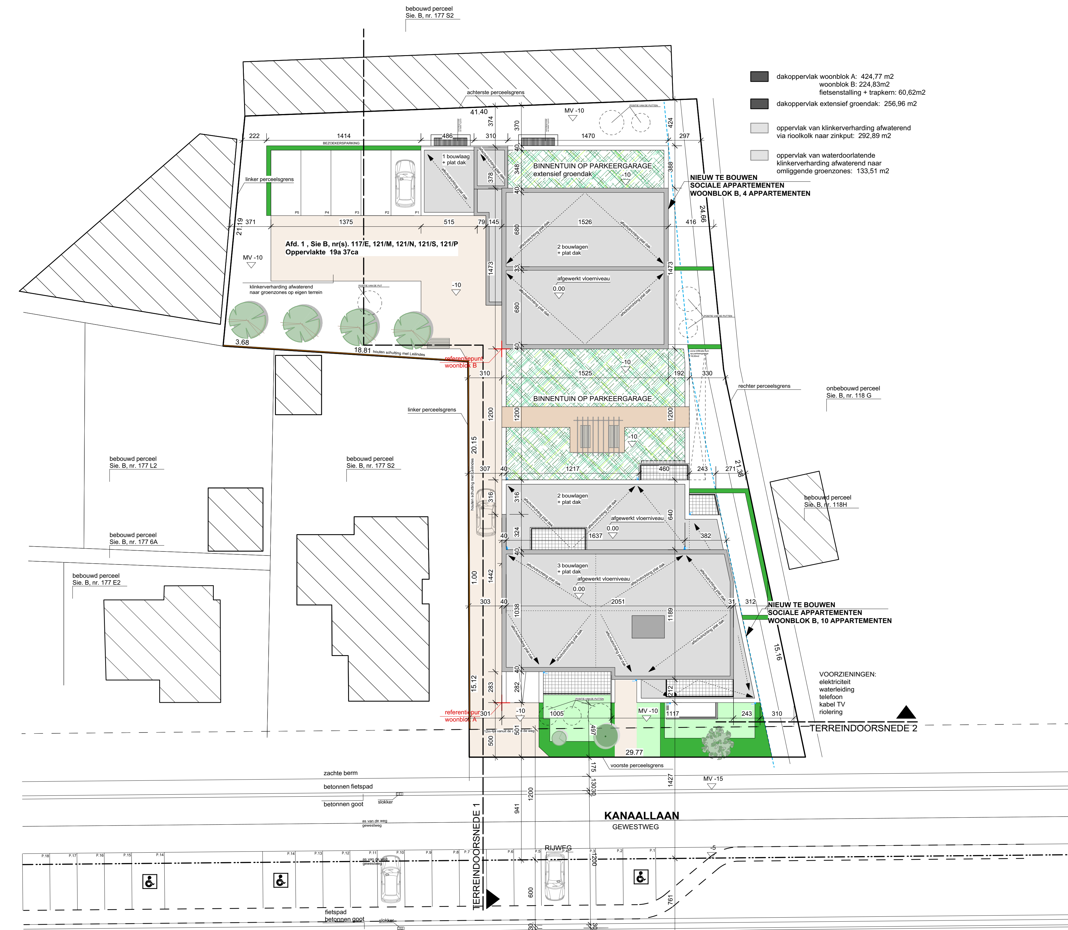
INPLANTINGSPLAN nieuwe toestand schaal 1/200
