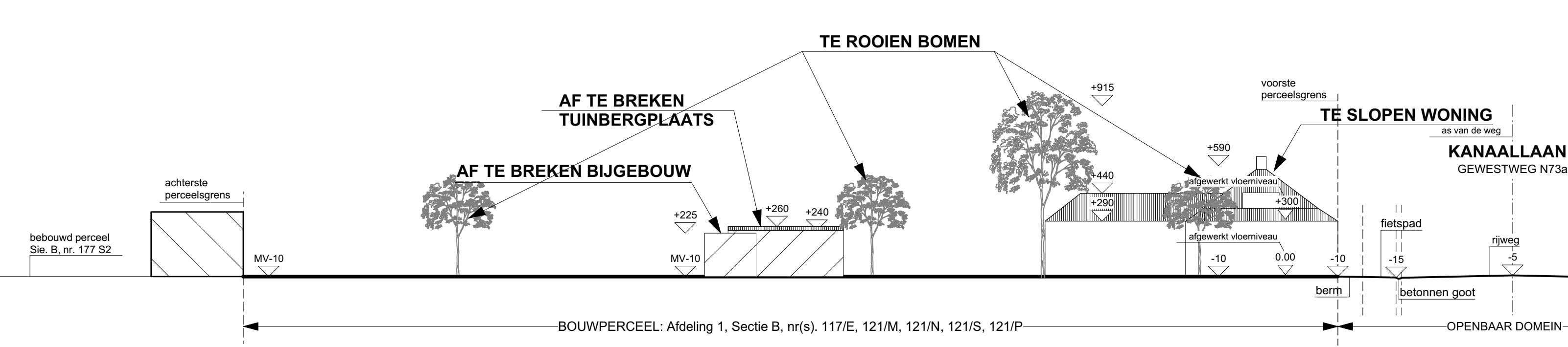
TERREINDOORSNEDEN 1 bestaande toestand schaal 1/200
