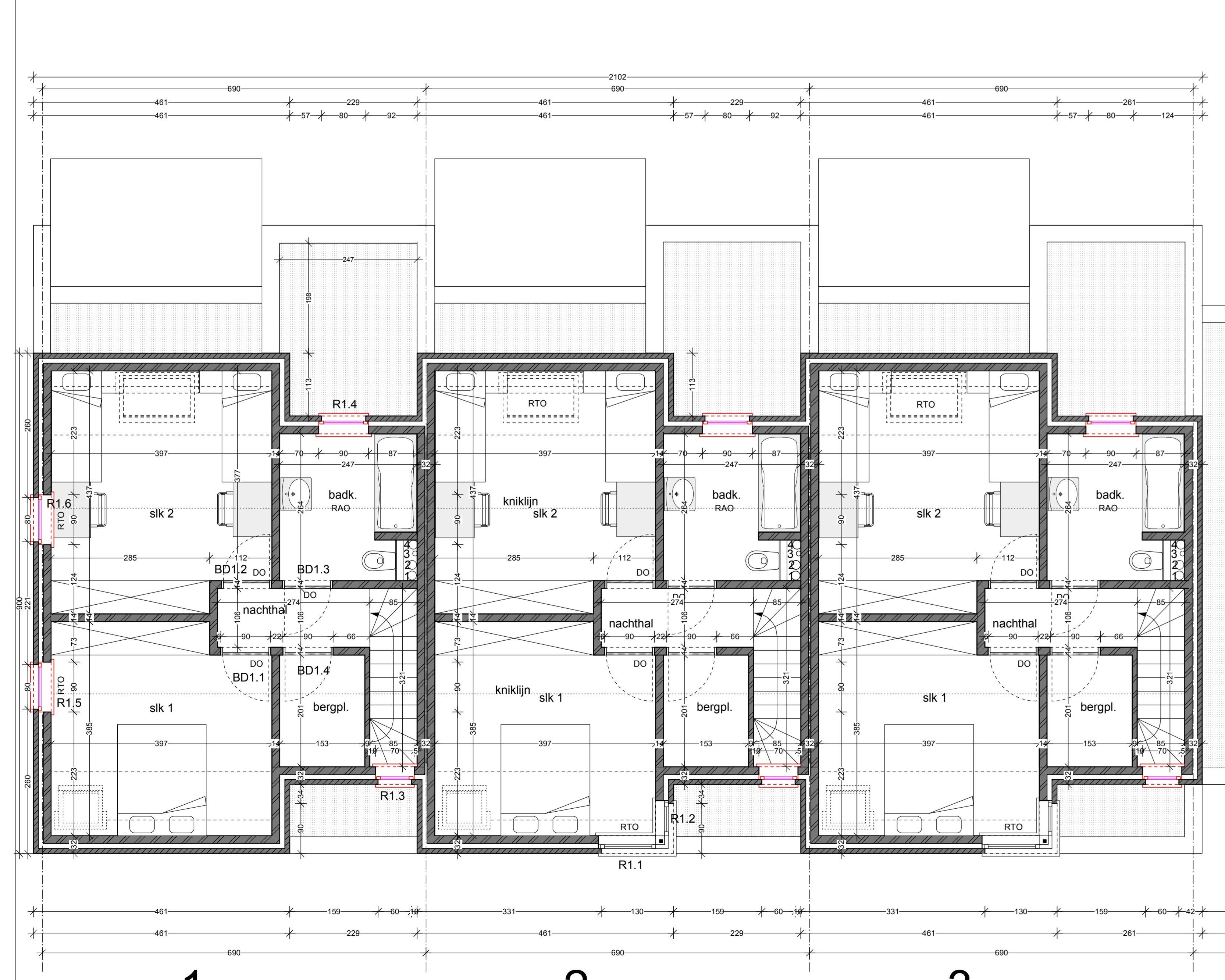
verdiepingsplan
