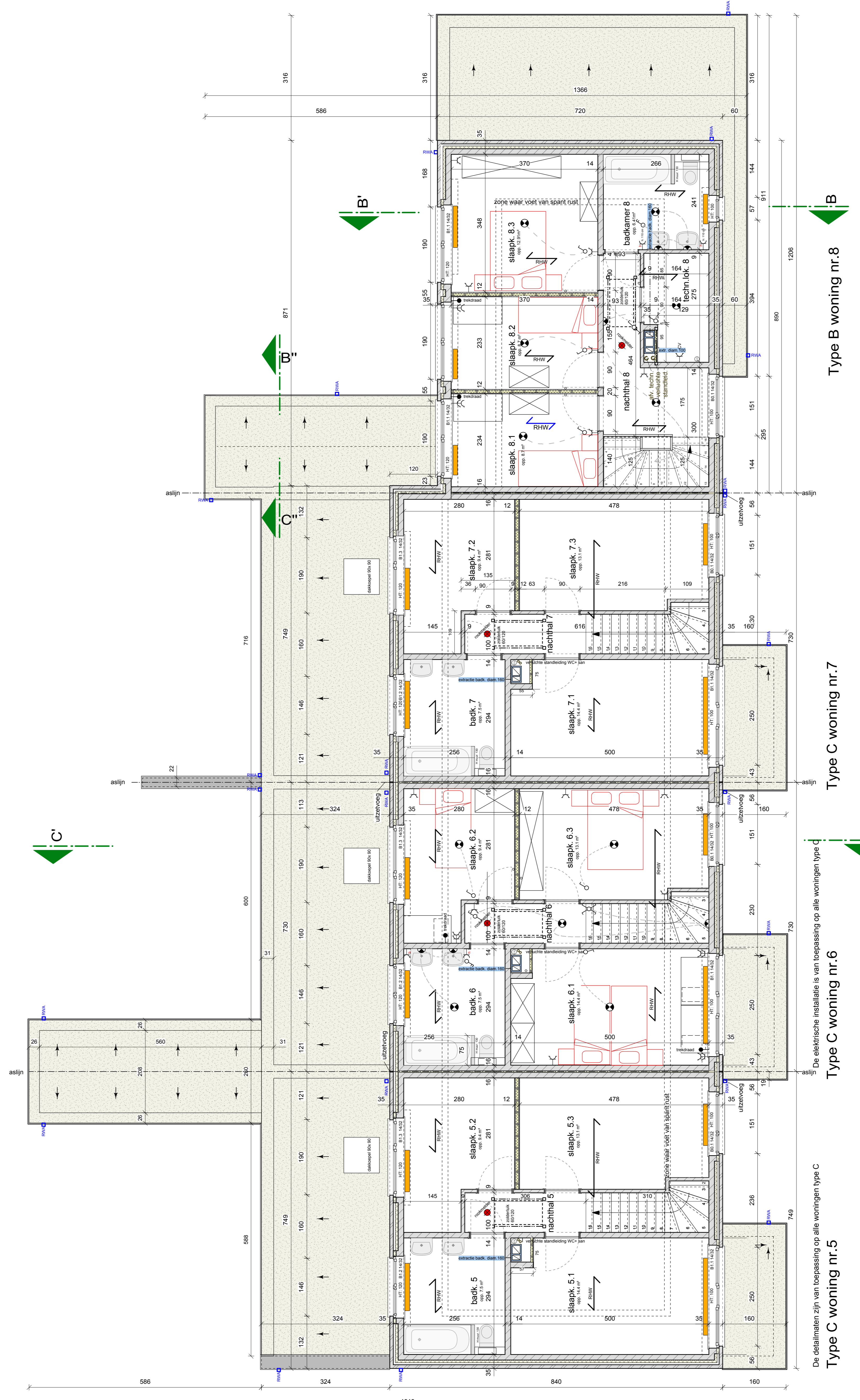
Eerste verdiep- schaal 1/50
