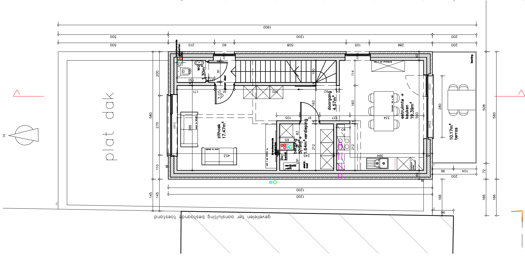
blok A. app. 2 : verd 1+2 type 3/4 4.21+56.02 +56.02=116.25m 2 1e VERDIEPING
