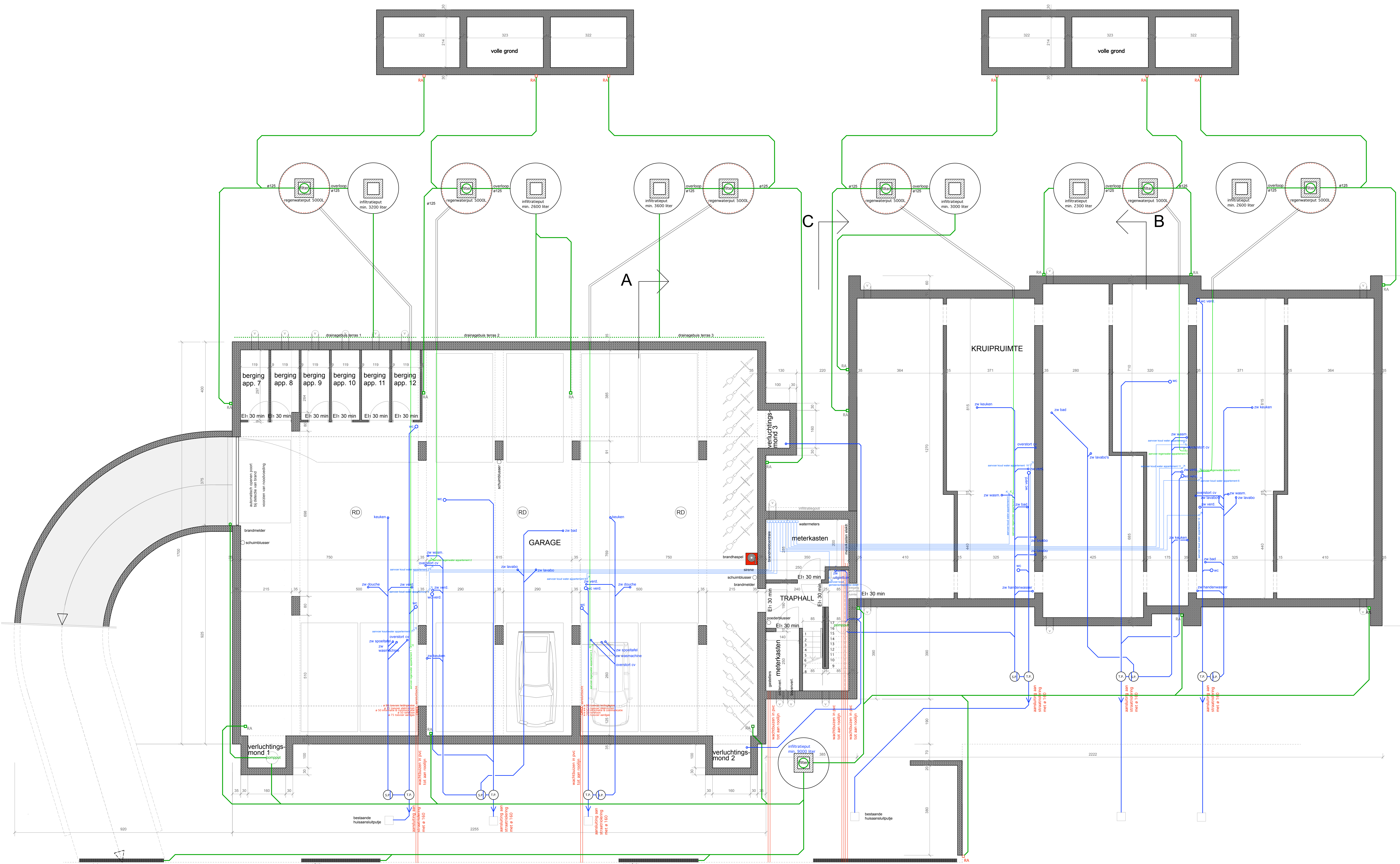
PLAN FUNDERING EN ONDERGRONDS GARAGE
